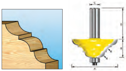
Frese: • = multiprofilo • = per smusso • = profilo classico
