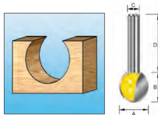
Fresa sferica
