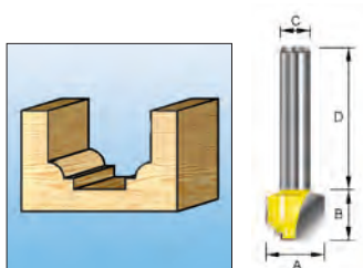
Fresa profilata
