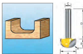
Fresa per cave 4R e 8R
