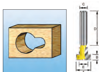
Fresa per foro serratura.
