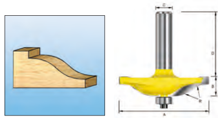
Fresa ad ogiva inclinata, non adatta a macchine con foro base minore di 75 mm.
