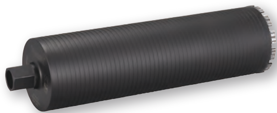
Attacco 1-1/4" UNC
