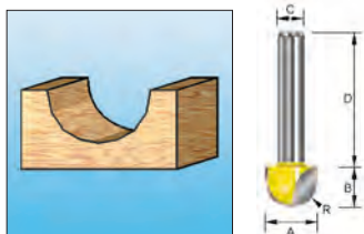
Fresa a raggio concavo
