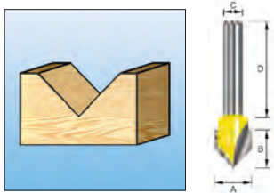
Fresa per scanalature a V
