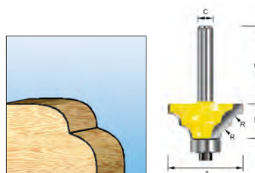
Fresa a doppio raggio
