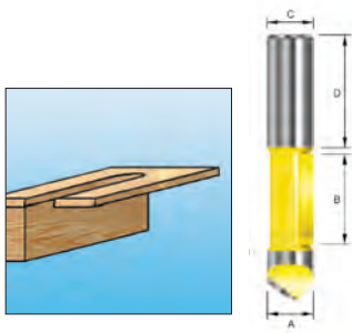
Fresa con guida
