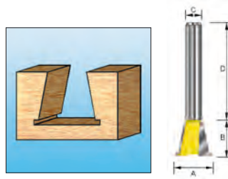
Fresa per incastri a coda di rondine
