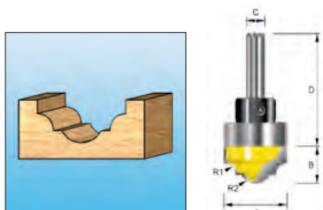
Fresa profilata
