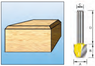
Fresa per rifilo e smusso
