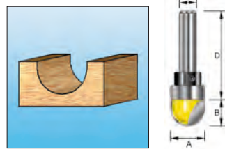
Fresa a raggio concavo
